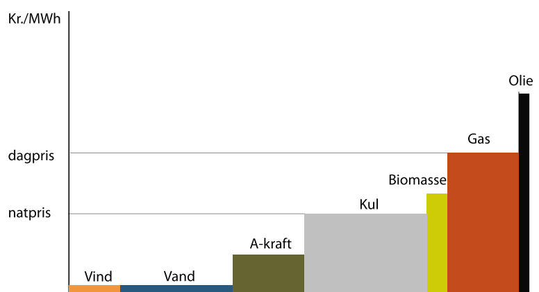
Stiliseret udbud-/efterspørgselskurve for det nordiske og tyske elmarked.
