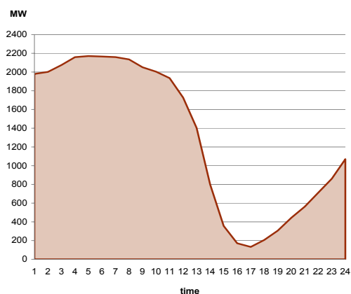
Vindkraftproduktion i Vestdanmark 8. januar 2005 under passage af stormen "Gudrun". Den maksimale reduktion time for time er 600 MW fra time 13 til time 14.
