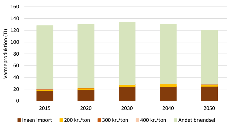
Figur 40: Udviklingen af fjernvarmeproduktionen i de forskellige scenarier, ved begrænsning på hvor meget overkapacitet der må være i systemet.
