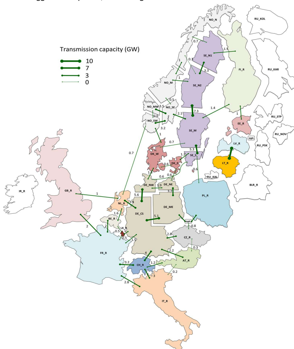
Figur 19: Geografisk dækningsområde for den regionale version af Balmorel. De angivne transmissionskapaciteter viser den tilgængelige kapacitet for markedet i 2015 (net transfer capacity). Mellem 2020 og 2030 er der i modellen medtaget etablering af Cobra kablet (Danmark-Holland) og VikingLink (Danmark-England).
