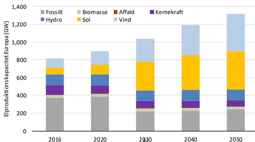
Figur 1: Fremskrivning af elproduktionskapaciteten i Nord-Vesteuropa. Fremskrivningen er udarbejdet med elmarkedsmodellen Balmore til dette projekt.
