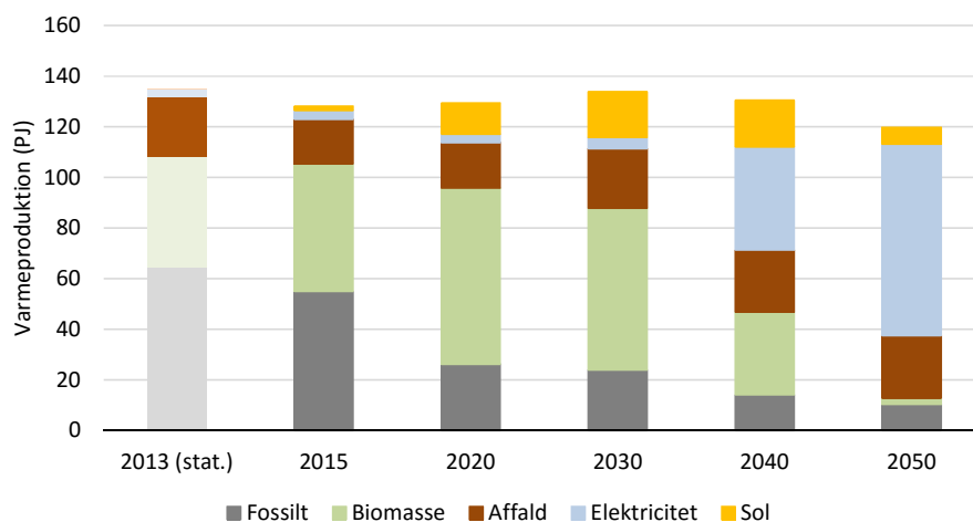
Figur 4: Udvikling af fjernvarmeproduktion i 'Ingen import' scenariet sammen med statistik for 2013 fra Energistyrelsens energistatistik 2014.
