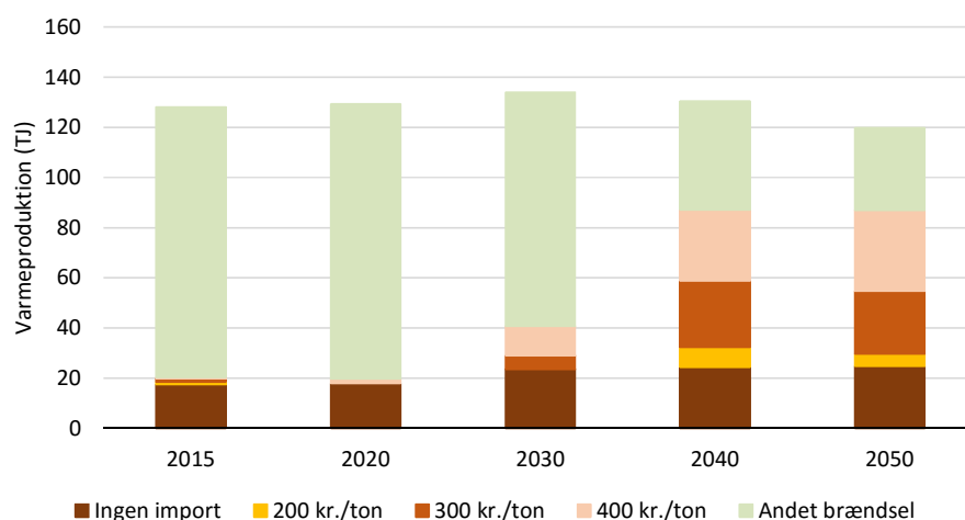
Figur 27: Udvikling af fjernvarmeproduktion i de forskellige scenarier.
