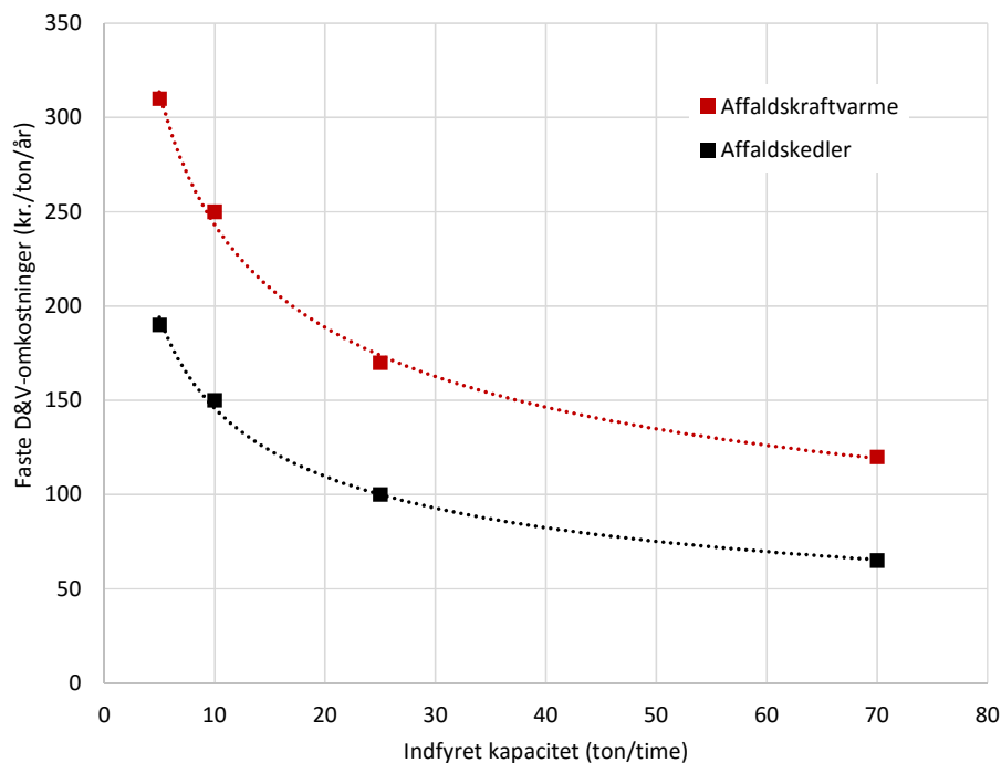
Figur 45: Fast D&V-omkostninger for affaldskraftvarme og affaldskedler afhængig af størrelsen på værket.
