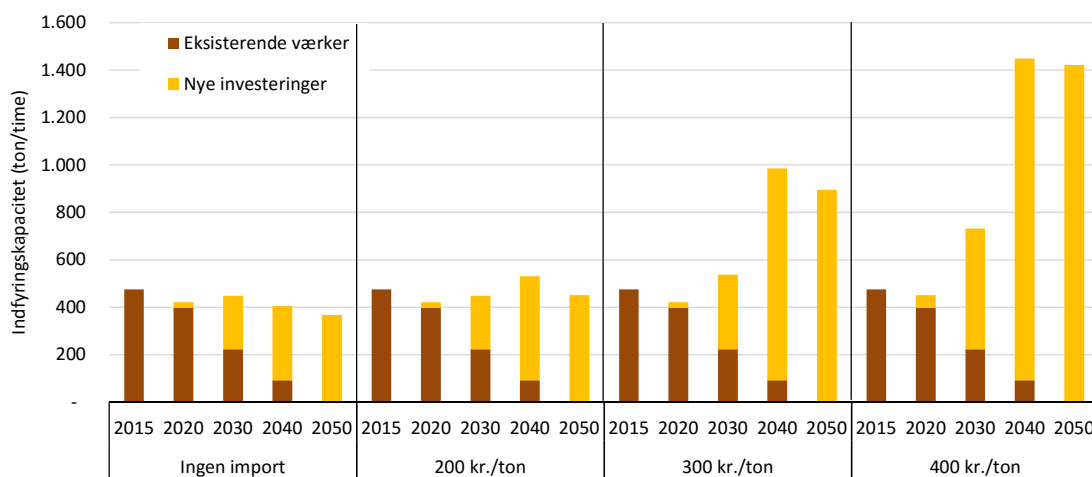
Figur 31: Udvikling i forbrændingskapacitet i de fire scenarier.
