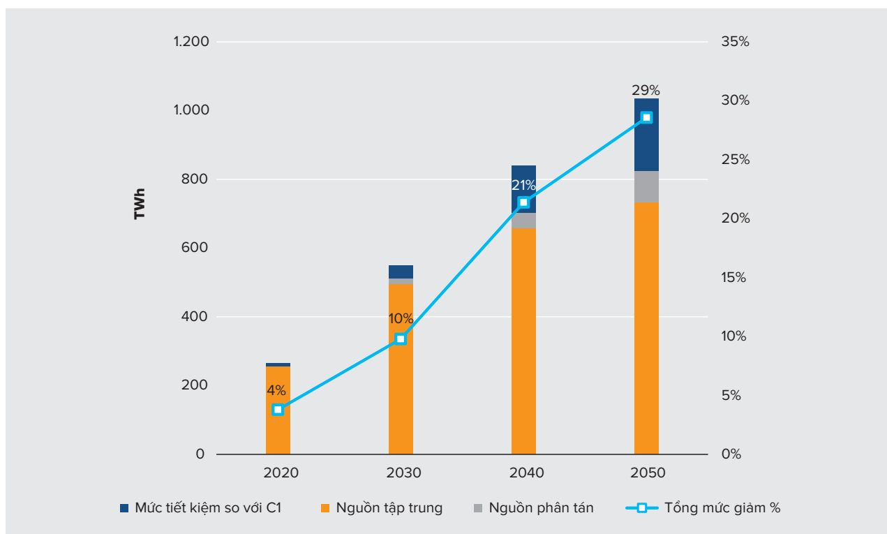
Hình 18: Các tác động của các biện pháp TKNL và các nhà máy nhiệt điện đồng phát trong công nghiệp trong Kịch bản C3 về TKNL so với Kịch bản C1 về Mục tiêu NLTT . Nguồn điện “phân tán” bao gồm xấp xỉ 80% là các nhà máy nhiệt điện đồng phát trong công nghiệp và 20% là điện mặt trời phân tán.
