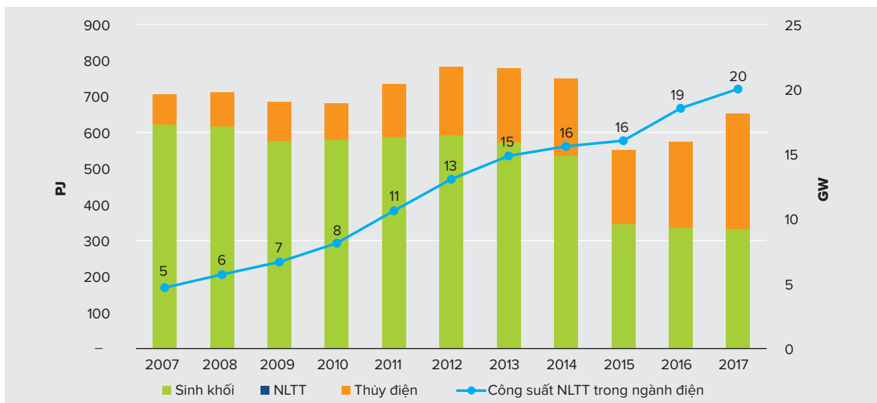
Hình 21: Phát triển NLTT (TPES) ở Việt Nam trong giai đoạn 2007-2017 (trục bên trái) và công suất điện NLTT (trục bên phải), trong đó bao gồm thủy điện nhỏ và lớn. Cần lưu ý rằng có sự thay đổi về công suất từ năm 2014 sang năm 2015 của nguồn cung sinh khối, một phần do sự thay đổi về phương pháp thu thập dữ liệu. Số liệu NLTT (TPES) cho giai đoạn 2007-2014 dựa trên (Viện Năng lượng, 2017) và giai đoạn 2015-2017 dựa trên (GSO, 2019), trong khi đó số liệu về công suất NLTT dựa trên (NLDC, 2018).
